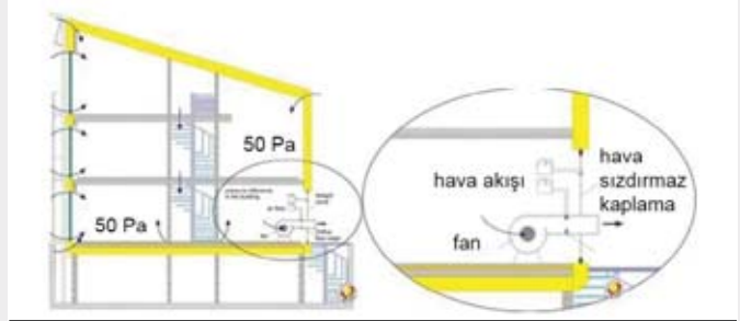
ŞEKİL 1.4 - PASİF EV KESİTİNDE BLOWER DOOR TESTİ PRENSİBİNİN GÖSTERİMİ
