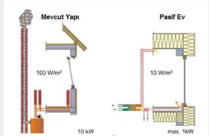
ŞEKİL 1.1 - PASİF EV VE GELENEKSEL EV TİPİNDE GEREKLİ MAKSİMUM ISITMA YÜKÜ
